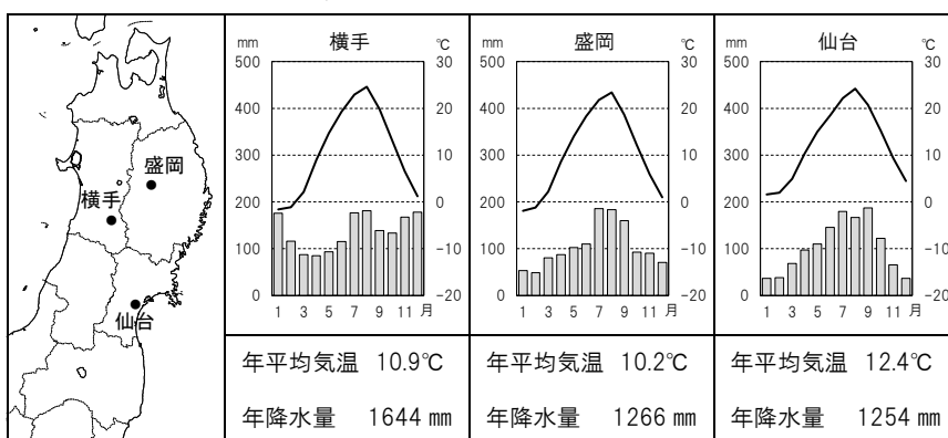
＜東北地方の主な都市の雨温図＞
